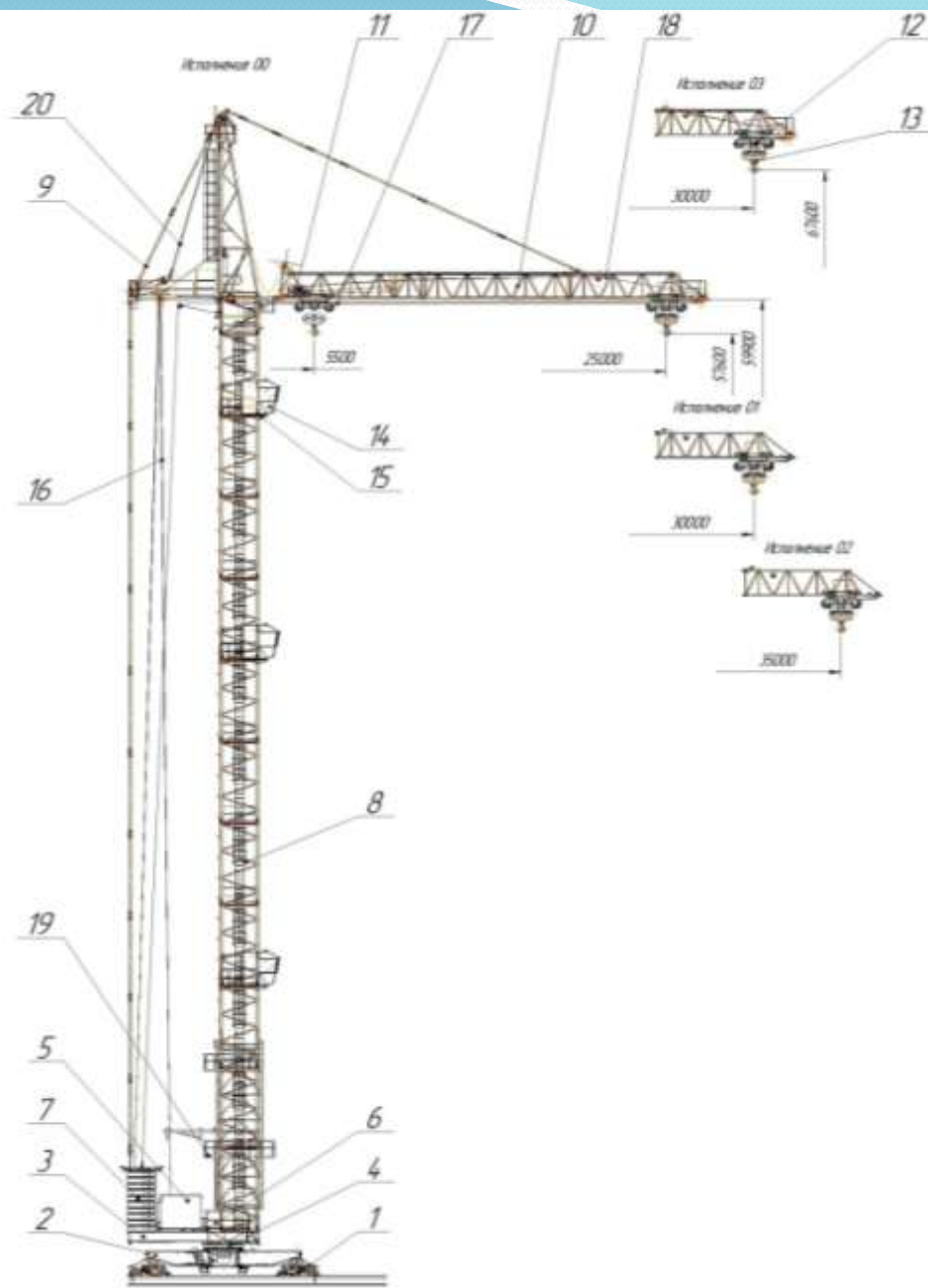
Рис.1 Башенный кран КБ-605
