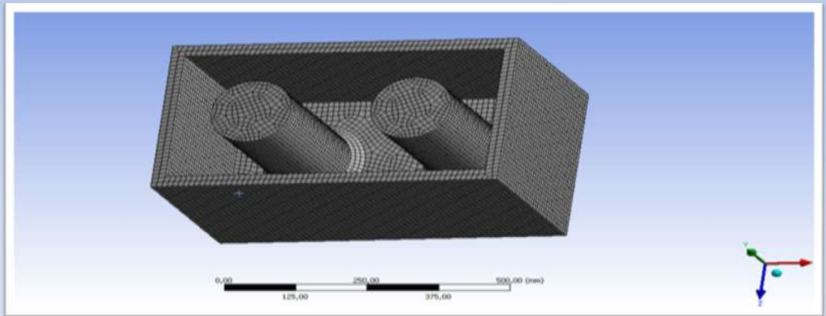
Конечно-элементное разбиение
